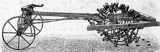
Рис. 2. Картофелесажалка.
