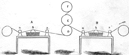
Рис. 8. Схема производства вулканизации двойной прокладываемой ткани по Паркеру.
