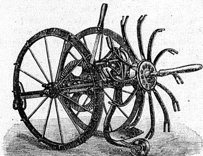
Рис. 5. Картофелекопатель гр. Мюнстеръ.
