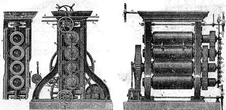
Рис. 5. Вальцы для получения пластинокъ каучука.
