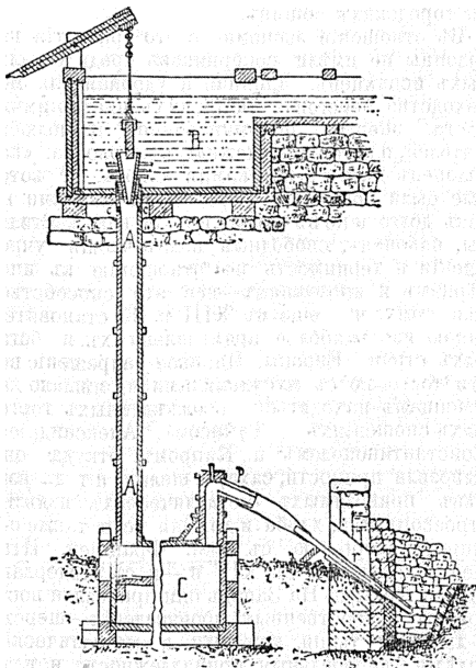
Каталонскій горнъ для полученія желѣза изъ руды, съ вододѣйствующимъ дутьемъ.
