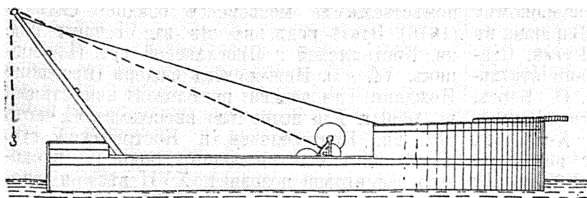
Фиг. 1. Карчеподъемный снарядъ, употребляемый на р. Донѣ.
