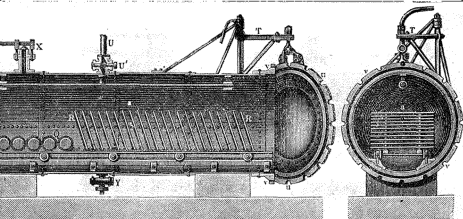
Рис. 2. Котелъ для вулканизации каучука (видъ съ боку и въ разрѣзѣ).
