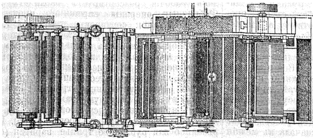
Цилиндрическая машина для производства картона: прод. разрѣзъ и планъ.
