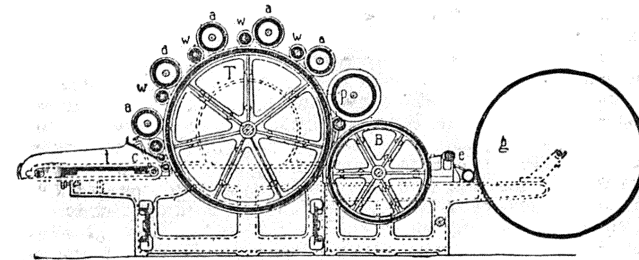
Фиг. 5. Кардная машина шерстопрядильная (въ продольномъ разрѣзѣ)
