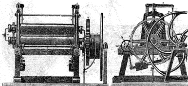
Рис. 1. Вальцы для промывания сырого каучука.
