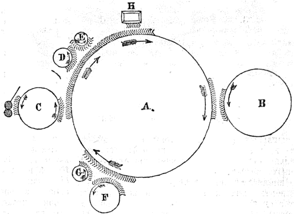
Фиг. 1. Схема расположенія главныхъ органовъ кардной машины.
