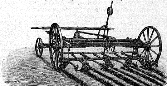
Рис. 6. Картофельный запашникъ.
