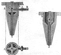
Рис. 6. Напечетникъ къ прессу для пригото- вленія каучуковыхъ трубокъ.
