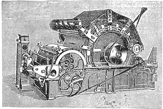
Фиг. 3. Кардная машина бумагопрядиель съ перемѣщающимися шляпками.
