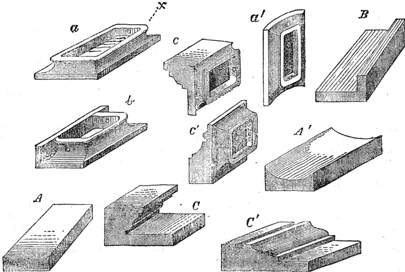
а, а', b, с, с'—печные изразцы для разныхъ частей печи. А, А', B, C, C'—формы или колодки, при помощи которыхъ изготовляются изразцы.
