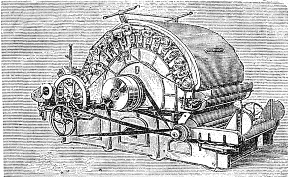
Фиг. 2. Валичная кардная машина бумагопрядельная.
