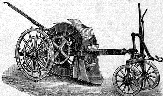
Рис. 10. Картофелекопатель «Paulus».
