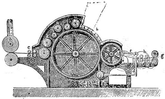
Фиг. 4. Кардная машина бумагопрядиель смѣшанной системы (въ продол. разрѣзѣ).
