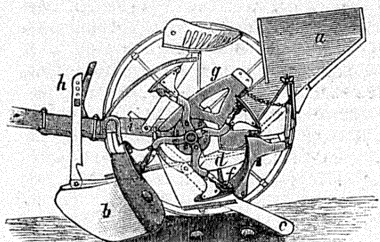
Рис. 1. Картофелекопатель Аспивала.
