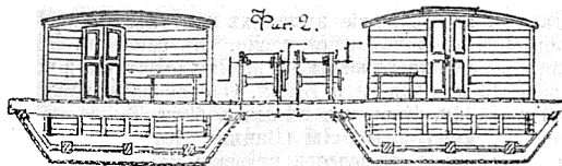
Фиг. 2. Карчеподъемница, употребляемая на рр. Днѣпрѣ и Березинѣ.
